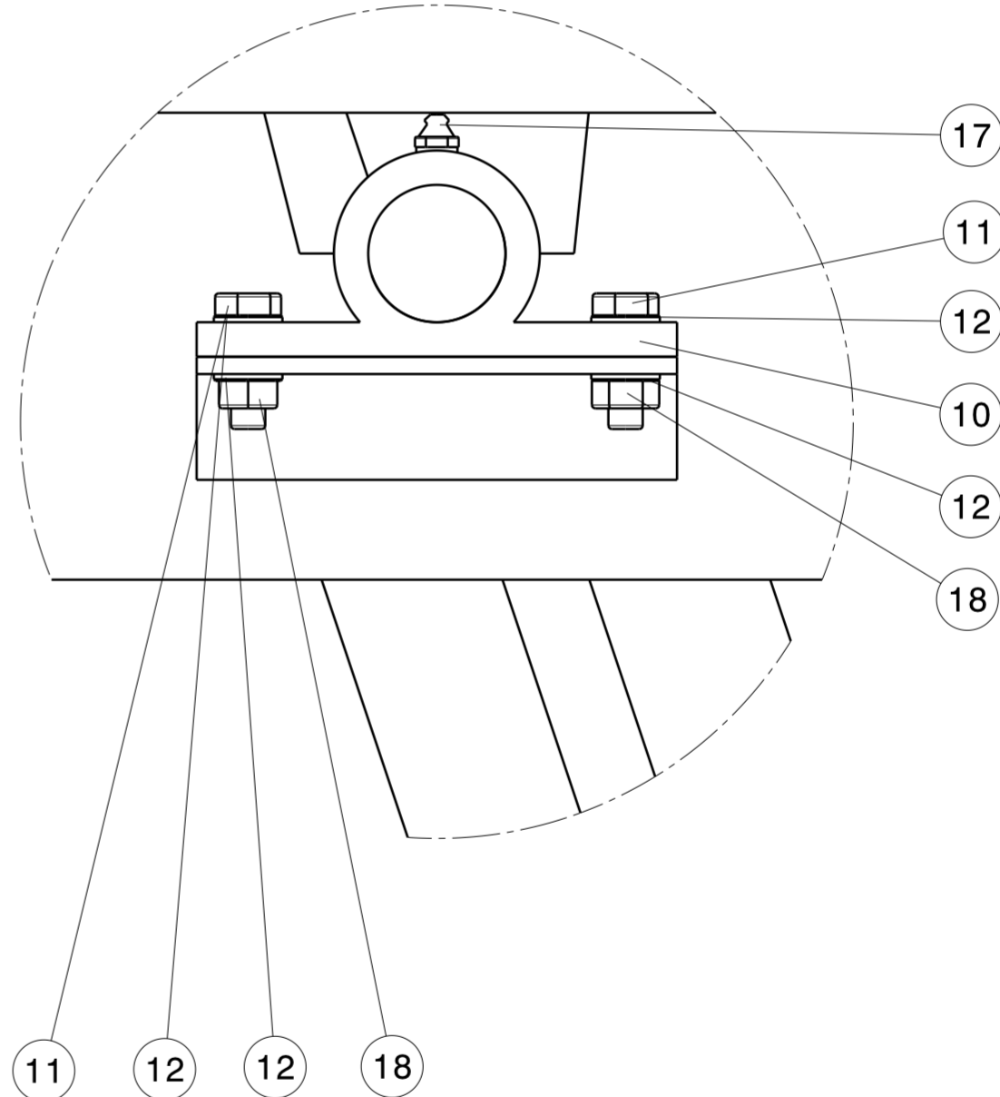
Detail B Maßstab: 1:2
